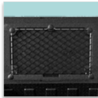
Filet pour plaques eutectiques ou glace carbonique
