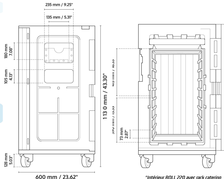
*Intérieur ROLL 220 avec rack catering
